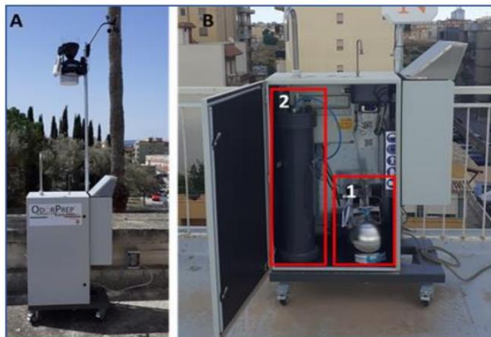
Centralina di campionamento – Chiusa (A); Aperta (B): 1. Canister; 2. sacca in nalophan™
