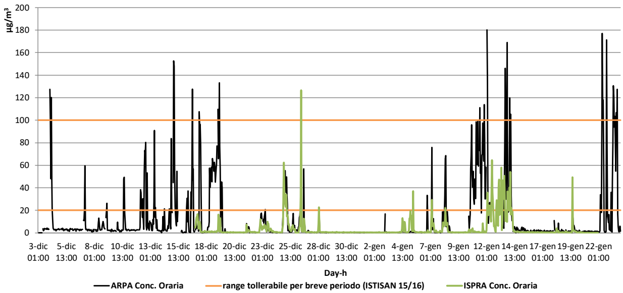
TREND H 2 S andamento orario (dal 3/12/2021 al 23/01/2022)
