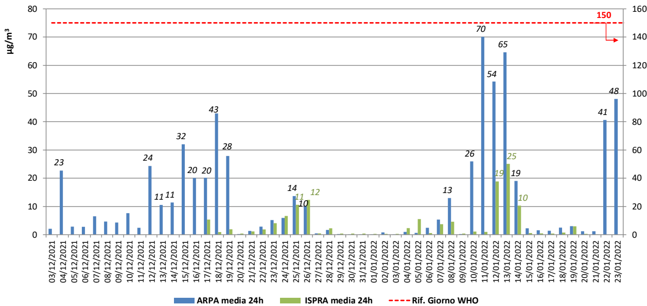
Trend H 2 S - Media giornaliera
