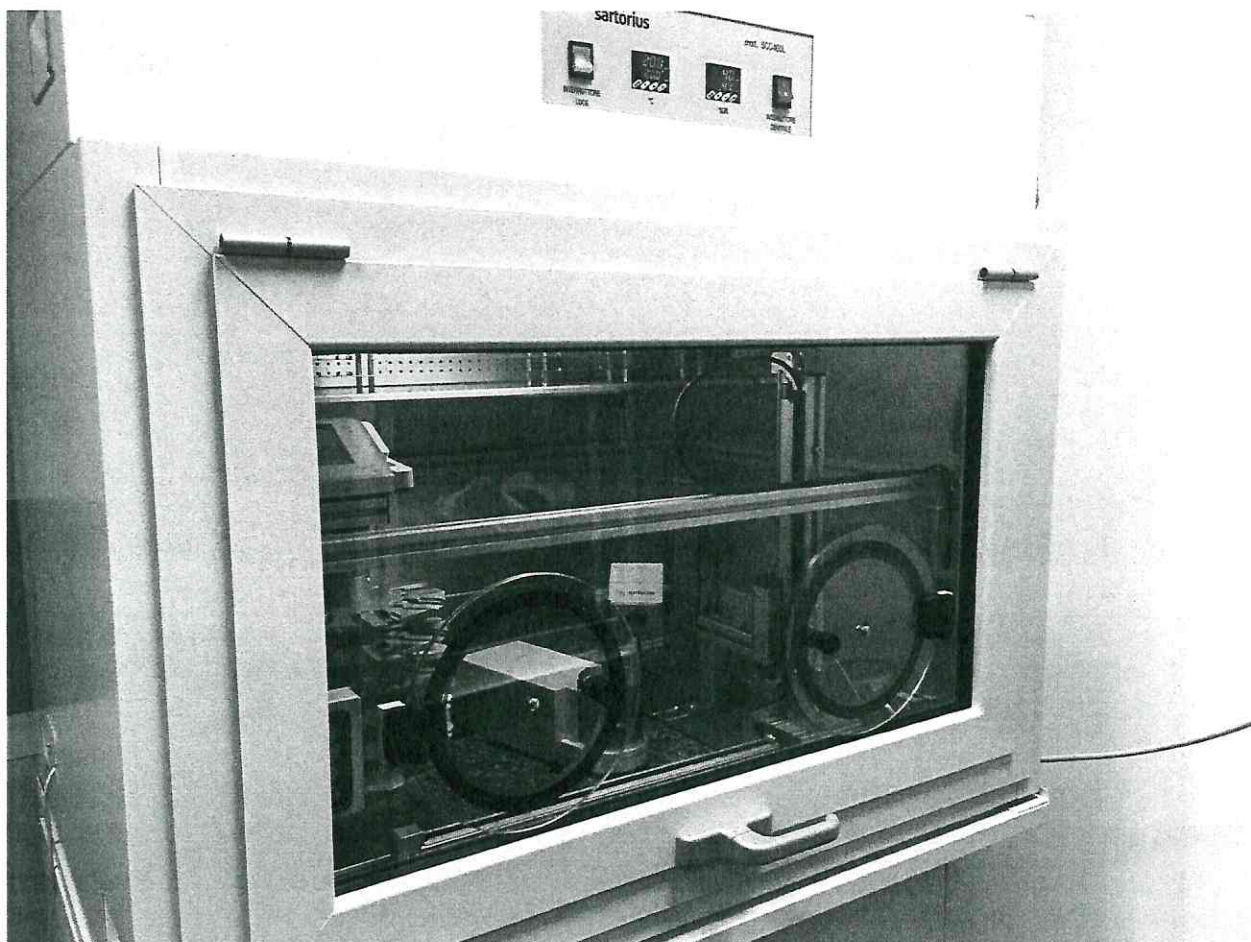
Fig. 5 Particolare della cappa climatica contenente il sistema robotizzato di pesatura, la bilancia di precisione, il tavolo antivibrante e gli accessori.
