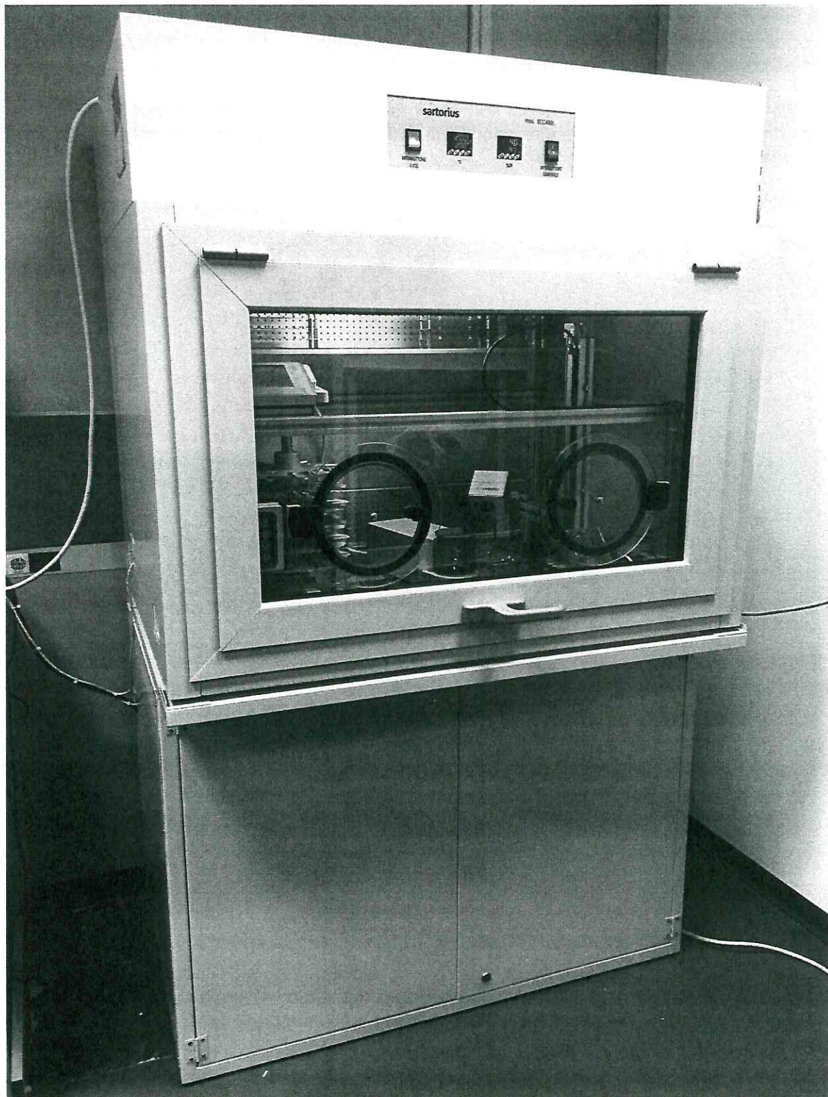
Fig 4. Sistema automatico per la pesatura dei filtri derivanti dal particolato atmosferico PM10 e PM2,5
