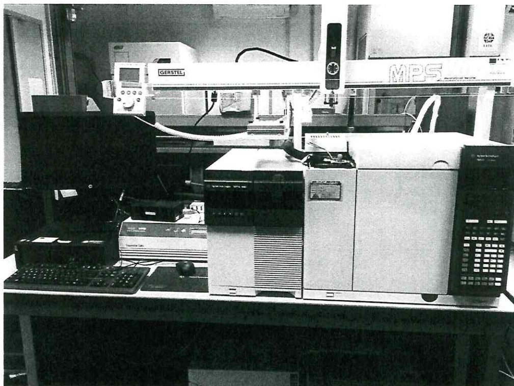
Fig. 1. Gas Cromatografo Agilent con rivelatore a spettrometro di massa completo di accessori.
