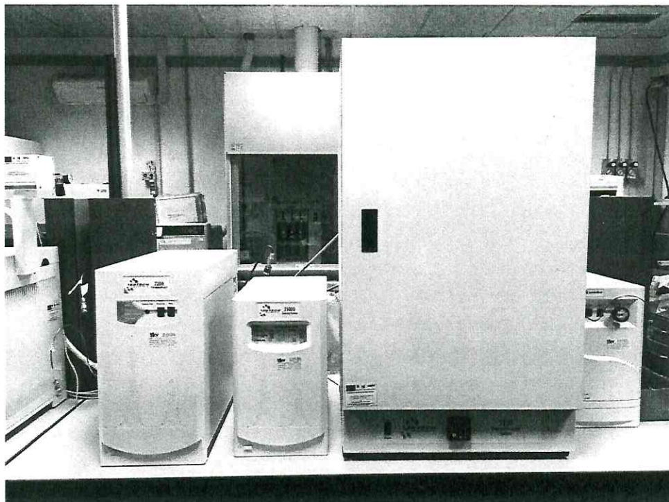
Fig 3. Linea di criofocalizzazione ad azoto liquido completa di accessori.
