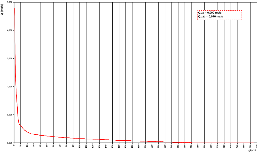
Curva delle durate Periodo storico 1970-1997 Periodo di osservazione 1974-1984; 1986; 1989-1990; 1992-1994
