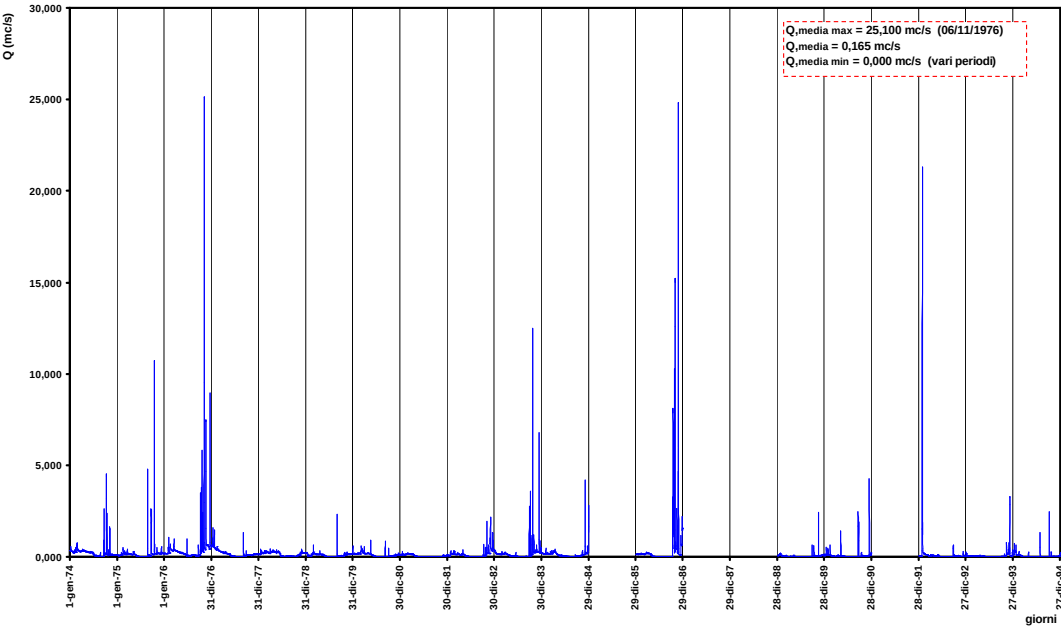
Portate medie giornaliere Periodo storico 1970-1997 Periodo di osservazione 1974-1984; 1986; 1989-1990; 1992-1994
