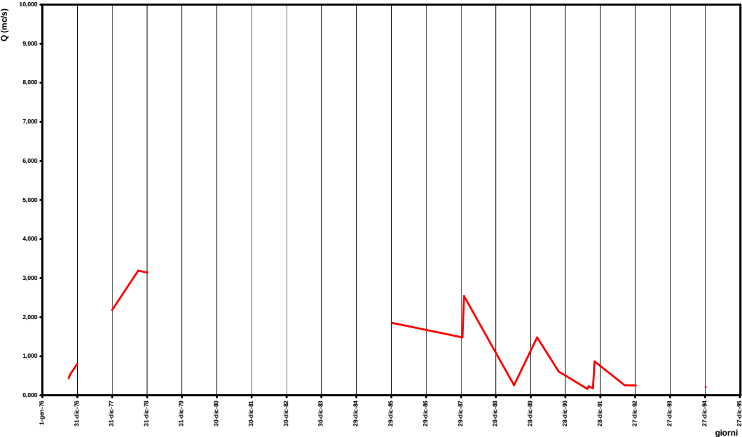
Deflusso di base Periodo storico 1970-1997 Periodo di osservazione 1976; 1978; 1986-1992; 1995
